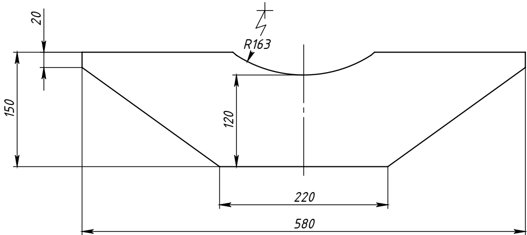
Поз.1 (Корпус) Развертка
