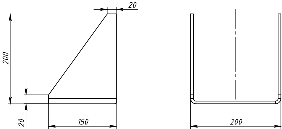
Поз.1 (Корпус)
